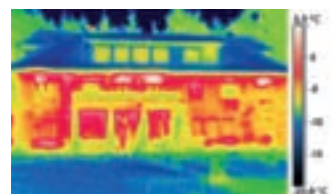
Thermografie direkt nach der ersten Bauphase: keinerlei Wärmeverluste durch das neu gedämmte Dach (blaue Färbung).
